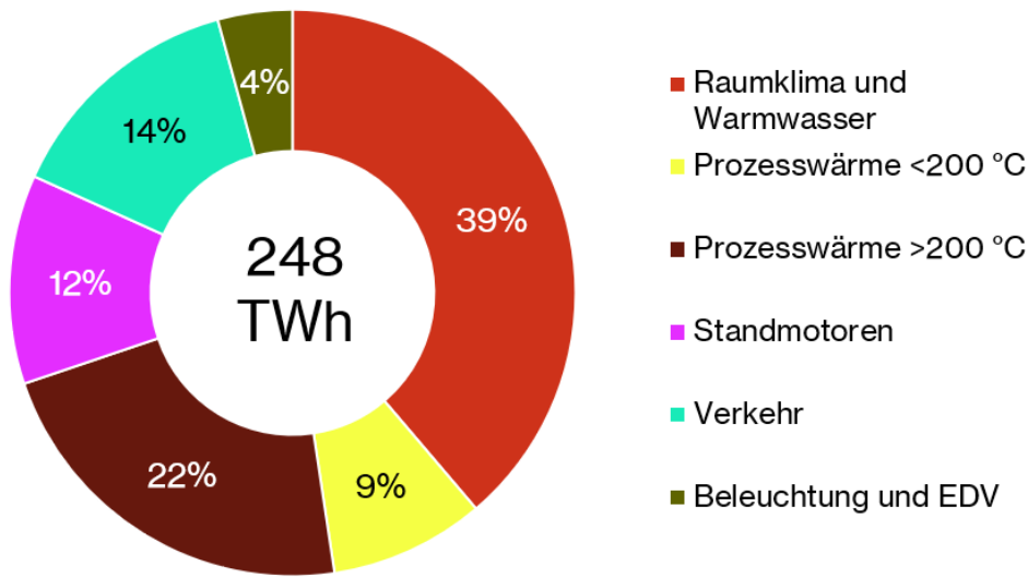
Abbildung 5: Endenergieverbrauch Österreich 2040 nach Nutzenergiekategorien
